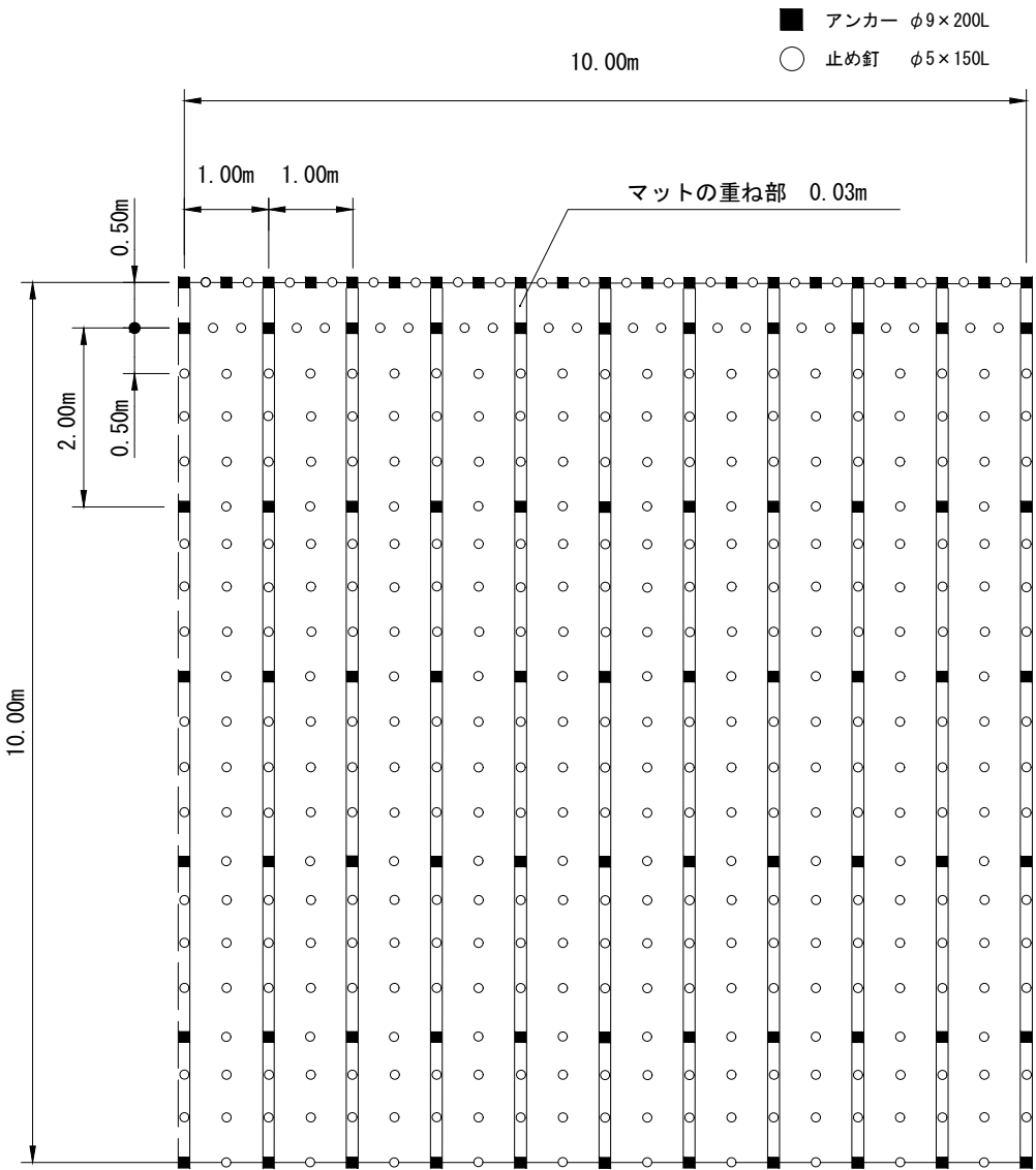
標準展開図
