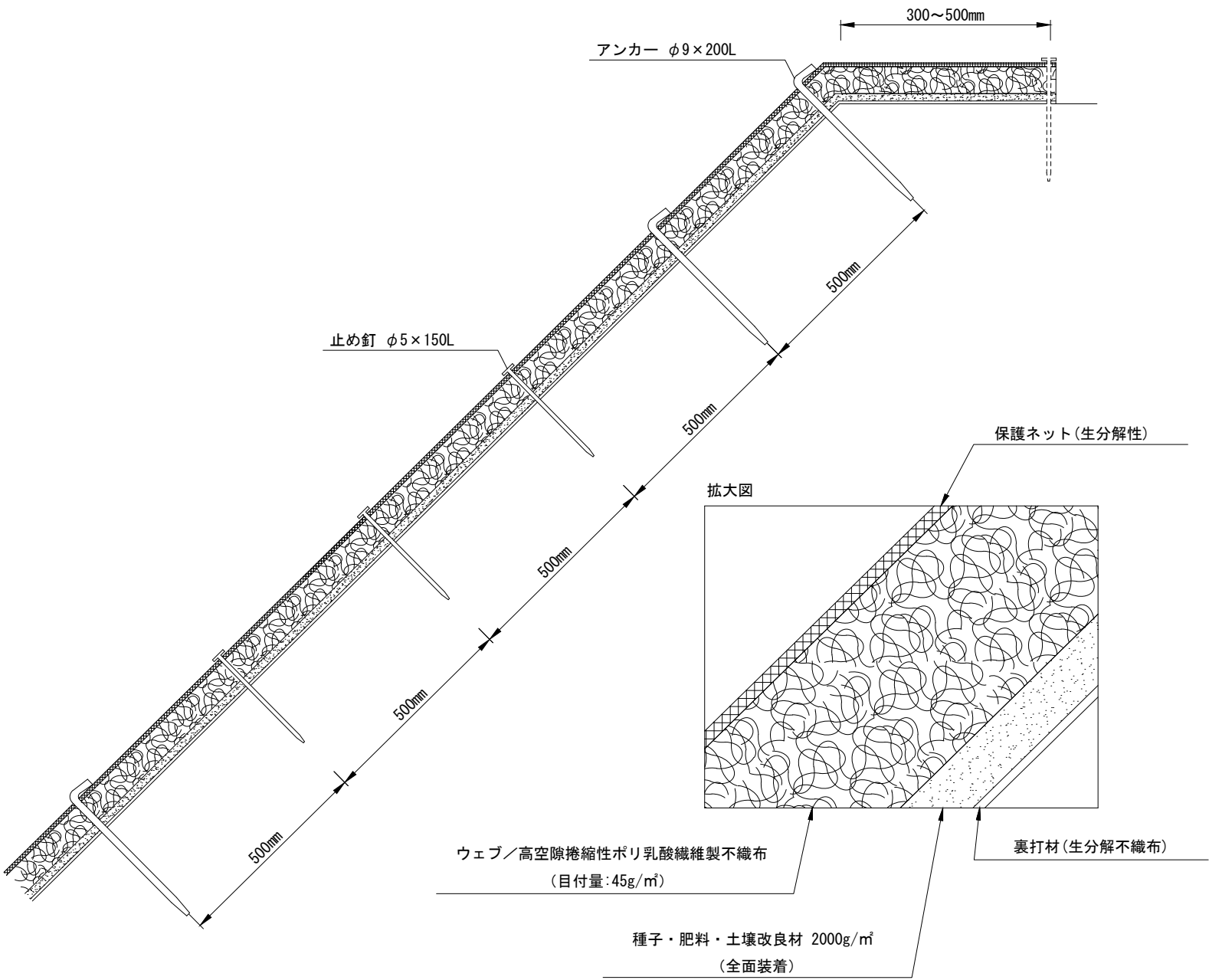
材料表 (100㎡当り)
