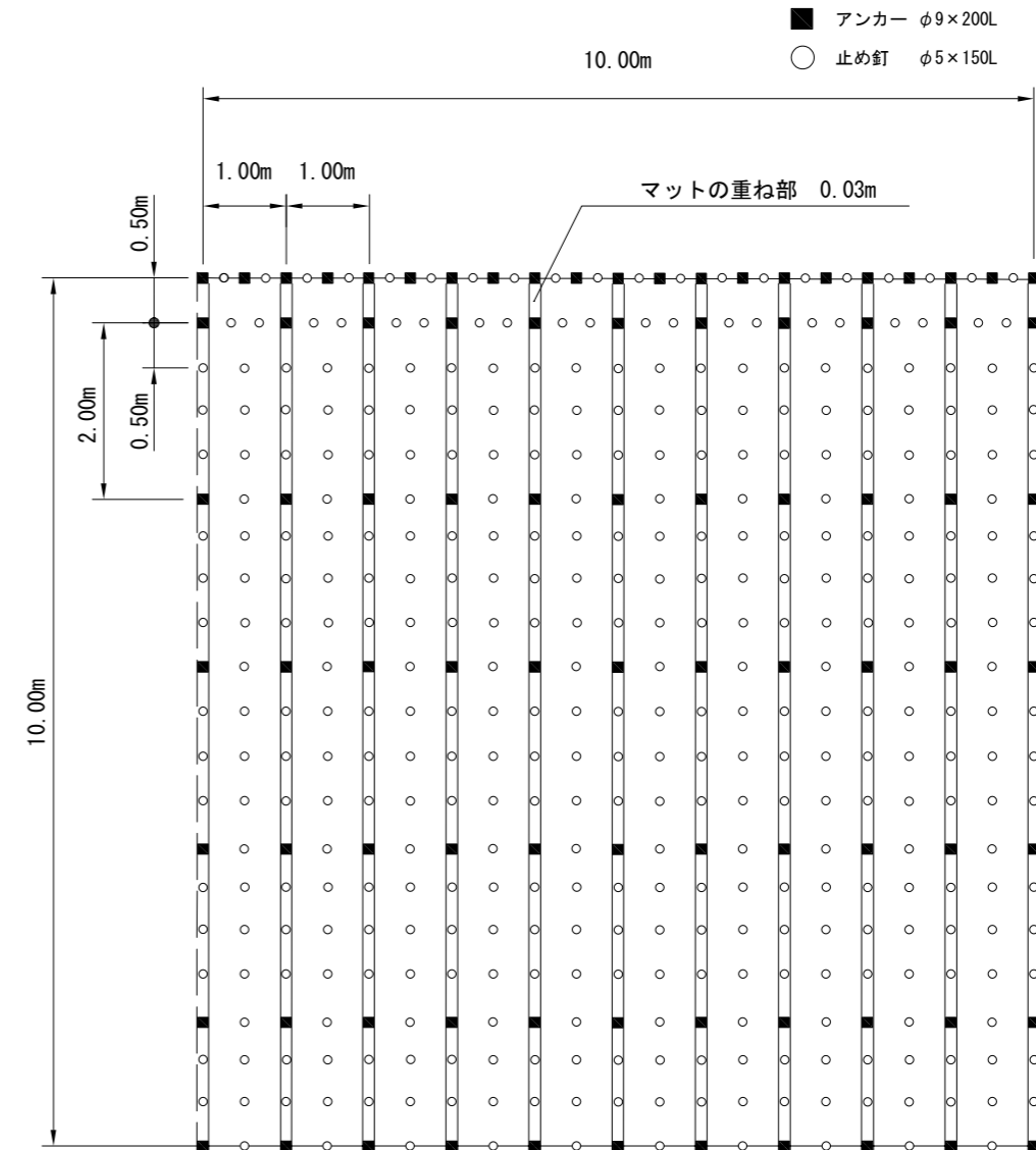
標準展開図
