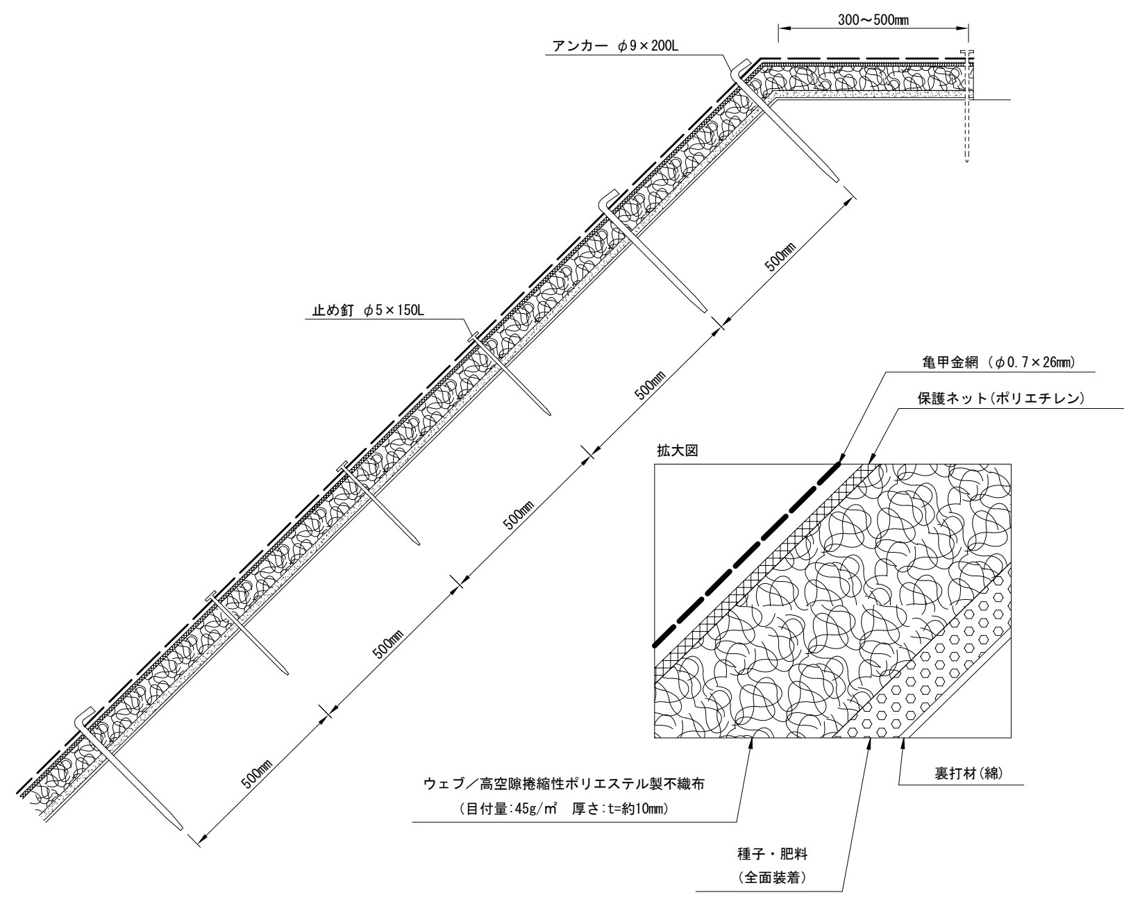
材料表 (100㎡当り)
