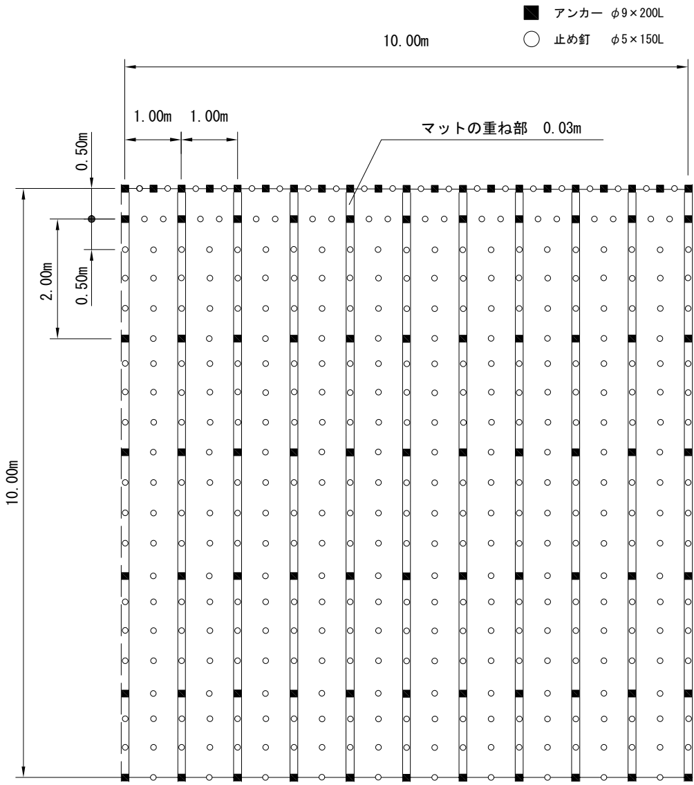
標準展開図
