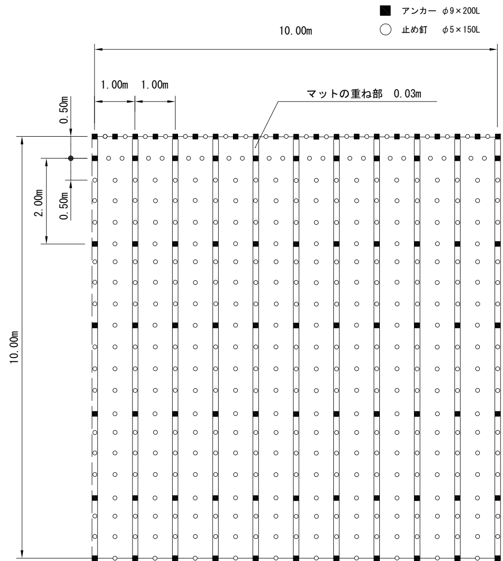
標準展開図
