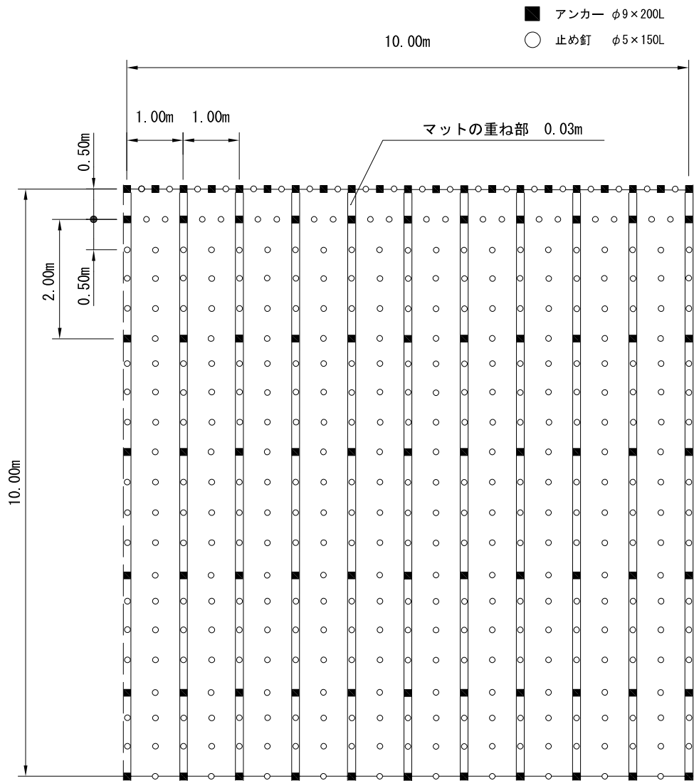
標準展開図
