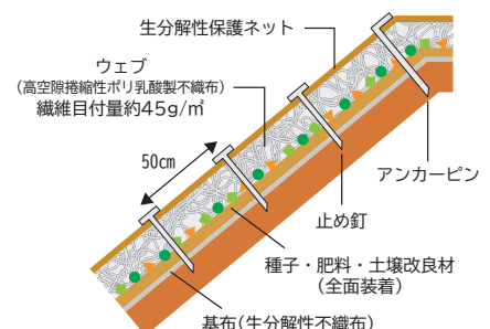
エコタイプ(種子・肥料有り、土壌改良材有り) 断面図/切土
