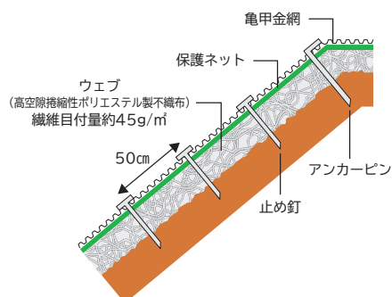
WNタイプ(種子・肥料無し、土壌改良材無し) 断面図/切土・盛土共通
