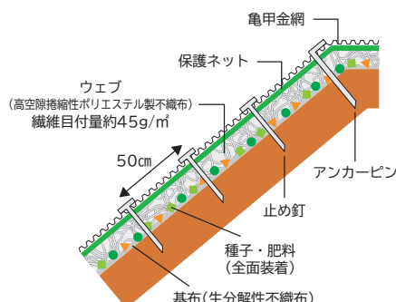
WNタイプ(種子・肥料有り、土壌改良材無し) 断面図/切土・盛土共通
