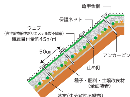
WNタイプ(種子・肥料有り、土壌改良材有り) 断面図/切土・盛土共通
