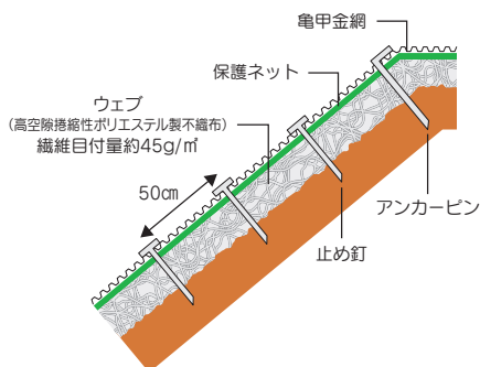
WNタイプ(種子・肥料無し、土壌改良材無し) 断面図/切土・盛土共通
